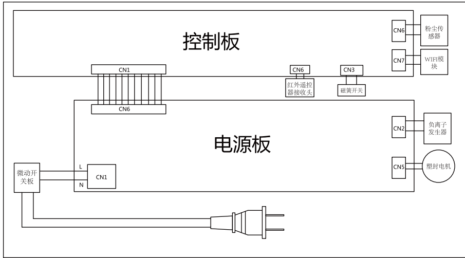
电气原理图
